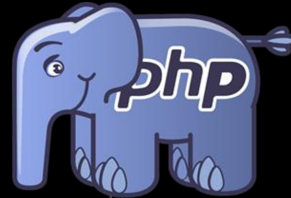
php
