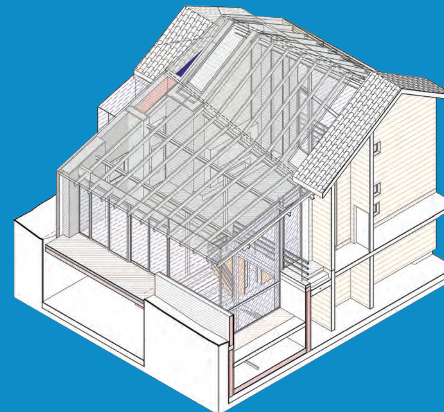
Рабочие 3д-схемы объекта
